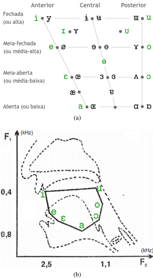
Fig. 1. Ilustração das posições das vogais no trapézio fonético e no gráfico F_1 \times F_2 . (a) Trapézio fonético das vogais de acordo com o IPA (International Phonetic Alphabet), com destaque em verde nas vogais que ocorrem no PB – reproduzido de [18]; (b) Sobreposição do gráfico de F_1 \times F_2 (eixos com valores decrescentes para facilitar a análise) e de uma ilustração com a posição da língua durante a produção das vogais orais tônicas – adaptado de [13].
